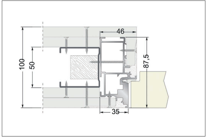
Çift alçı panel duvarlı kapı kasası Door frame with double plasterboard walls Duvar Kalınlığı 100 mm Door frame 100 mm
