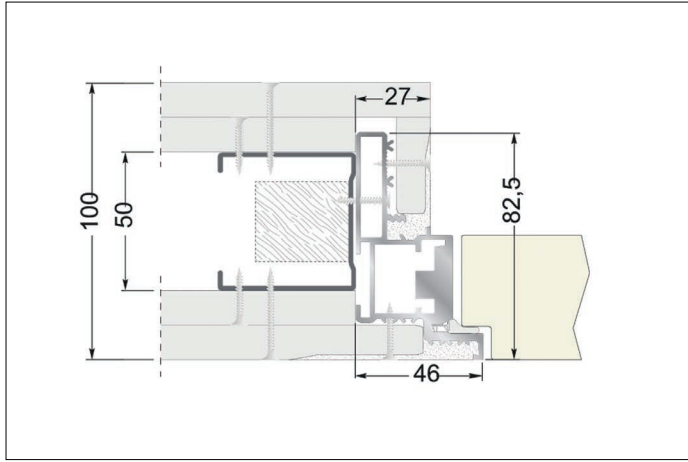
Çift alçı panel duvarlı kapı kasası Door frame with double plasterboard walls Duvar Kalınlığı 100 mm Door frame 100 mm
