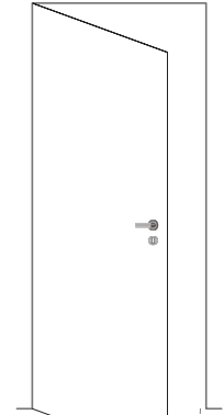
Çekme Uygulamalı Flush with wall on the pulling side
